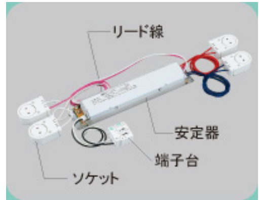
安定器ユニット
